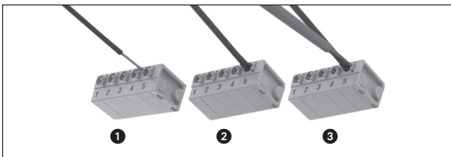
Abb. 2 Federkraftklemmen
