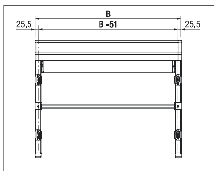
Montageplan B = Totalbreite
