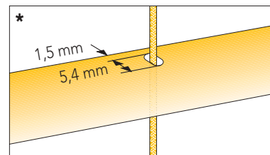
Nicht sichtbare Lamellenstanzung bei geschlossenen Lamellen.
