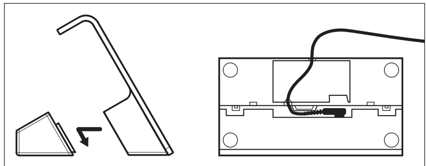
Abb. 1 Ladestation als Tischhalter
