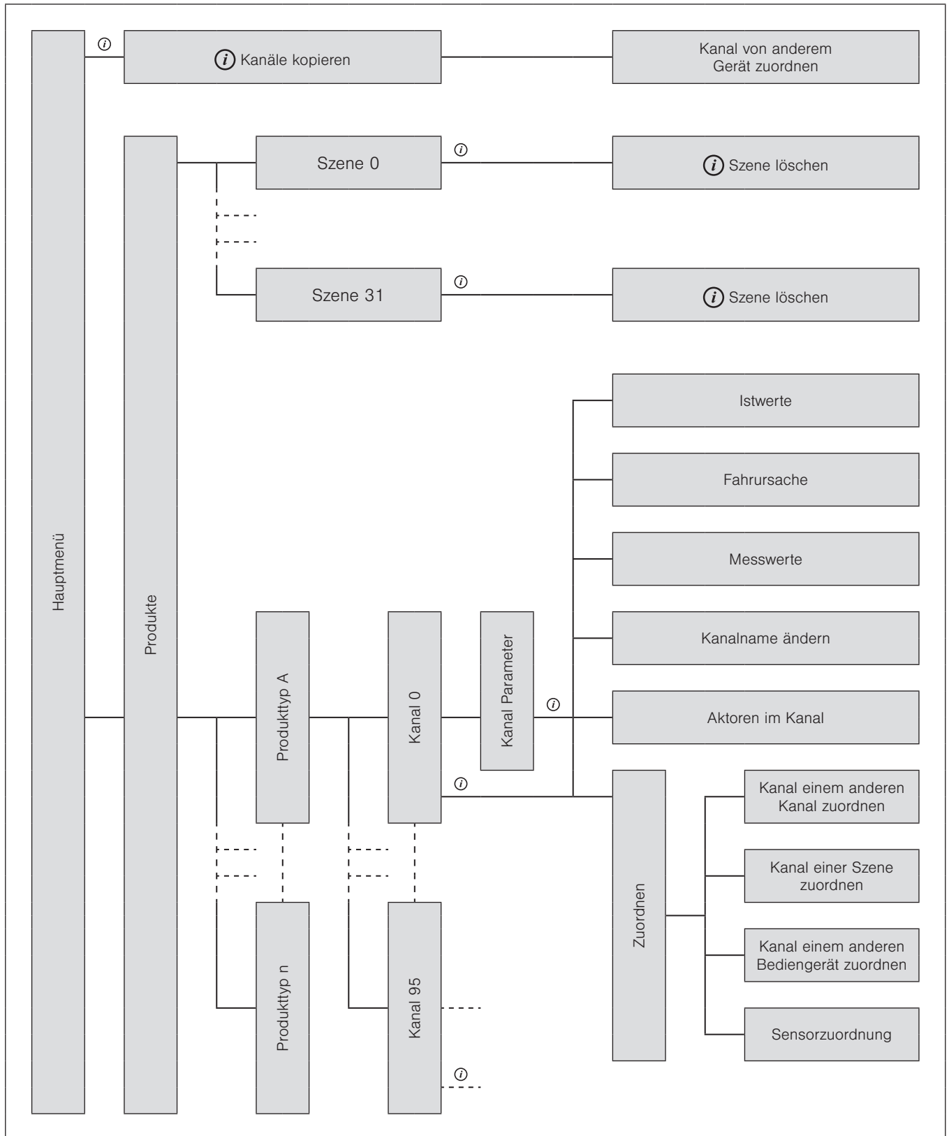
Abb. 12 Menü Produkte
