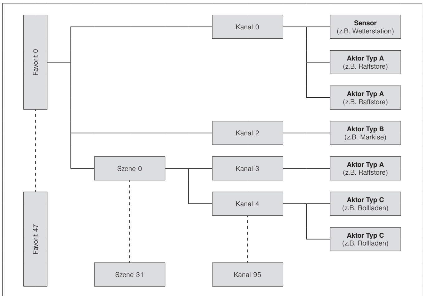
Abb. 10 Organisationsebenen
