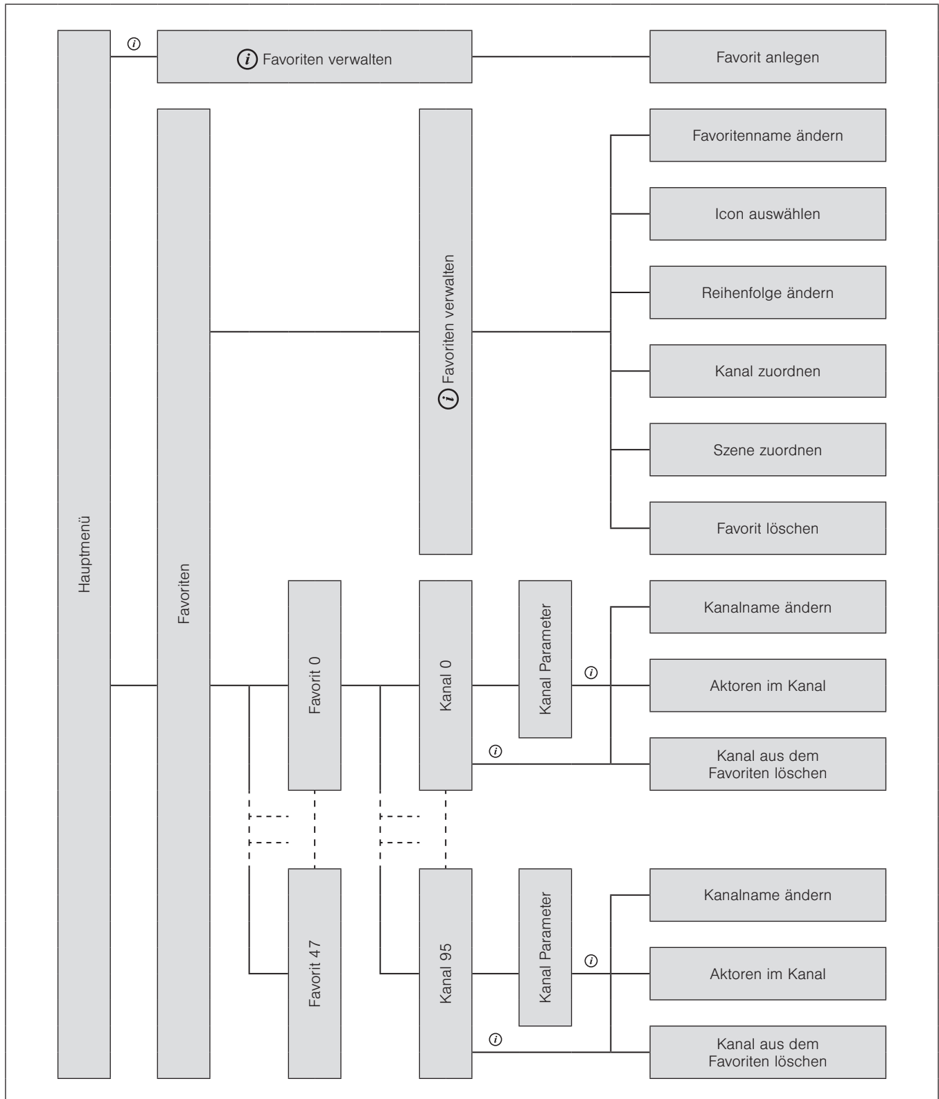
Abb. 11 Menüs Favoriten
