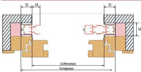
Anschlagprofil als seitliches Ausgleichprofil
