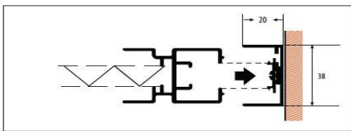
Anschlagprofil als seitliches Ausgleichprofil
