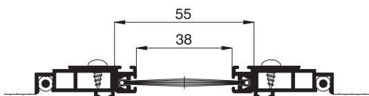
Schnitt A-A
