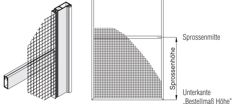
Bsp.: Sprosse SP6
