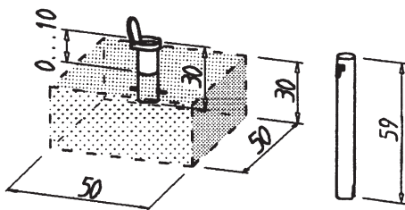
Bodenhülle mit Übergangrohr für Beton-Fundament
