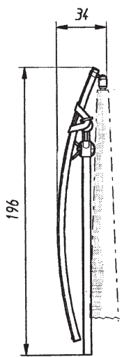
Alu-Gestänge 8.5 kg (Lift eingebaut 2.3 kg) (10.8 kg)
