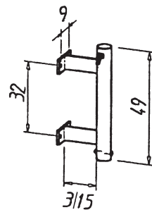
Wandbriden 3 oder 15 cm
