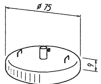
Betonsockel 90 kg
