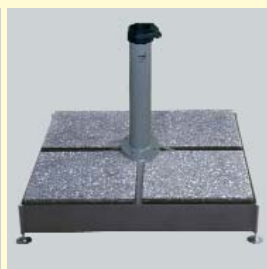
350 01 108 000 Schirmsockel grau pulverbeschichtet 350 01 207 160 Standrohr grau pulverbeschichtet 350 01 226 908 Gartenplatten 40 x 40 x 4 cm, 8 Stück (ca. 110 kg)
