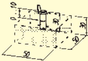
Bodenhülle mit Übergangrohr für Beton-Fundament
