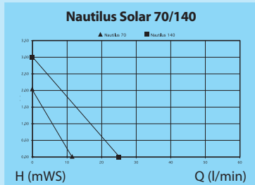
Pumpenkennlinie
